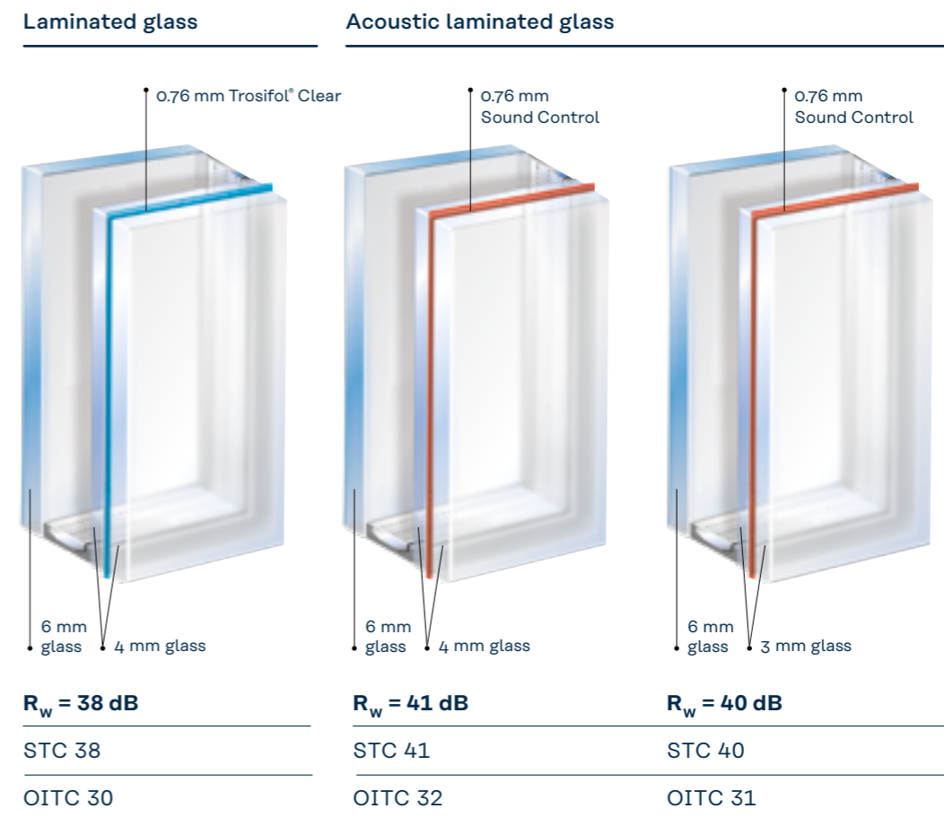
TAB 39 • 0.76 mm = 30 mil
